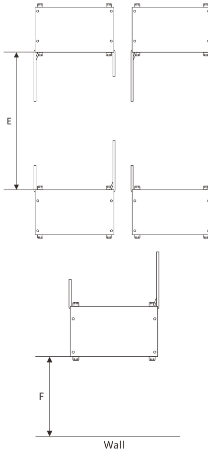
Zeichnung des Montagefreiraums (Draufsicht)
